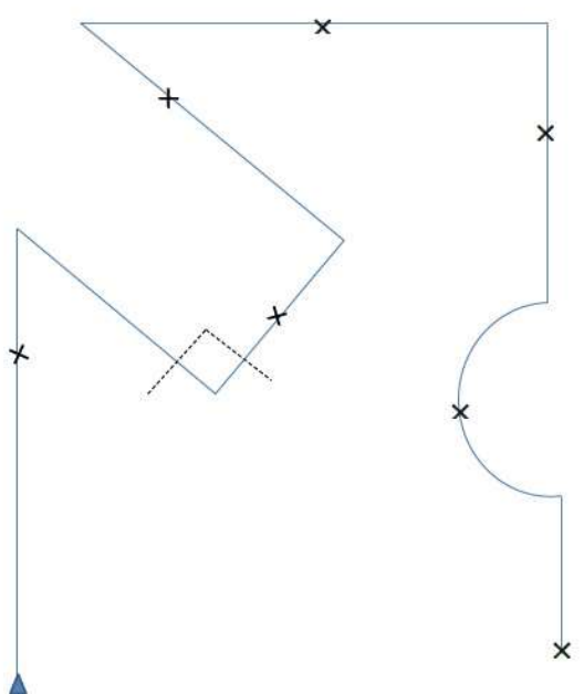
Obr.č.6 – Příklad tvarů stop IFH-2 (IGP-FH)
