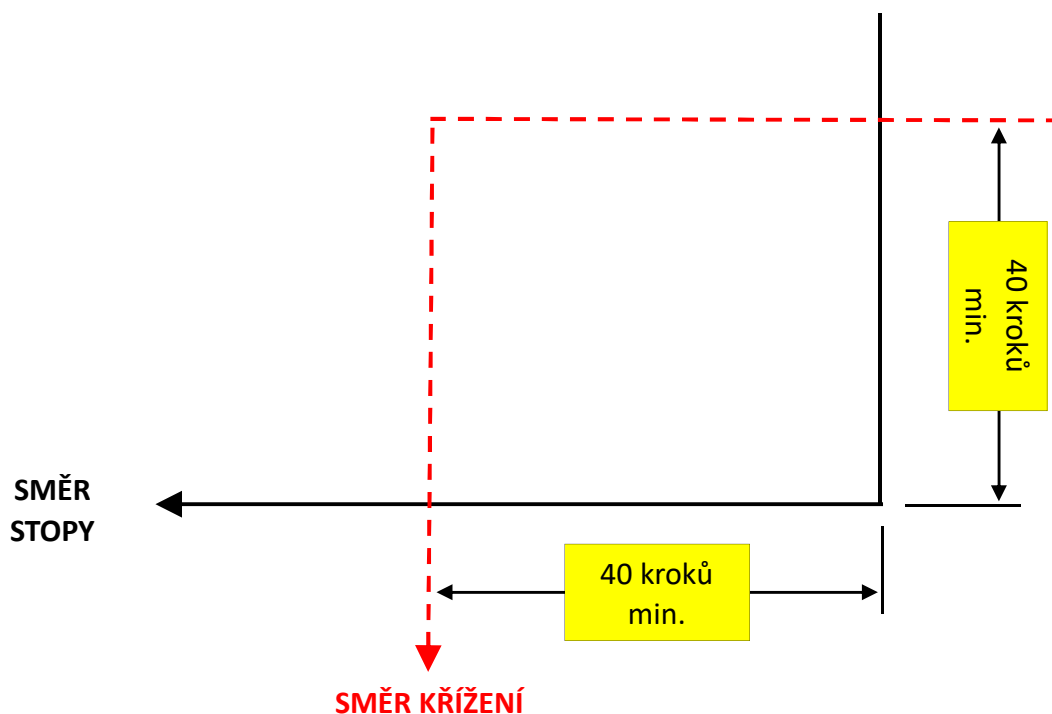
Obr.č.18 – křížení pravouhlého lomu
